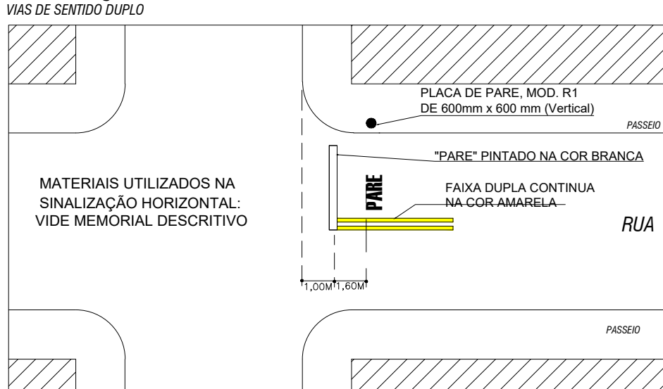
DETALHE - SINALIZAÇÃO DE PARADA OBRIGATÓRIA
