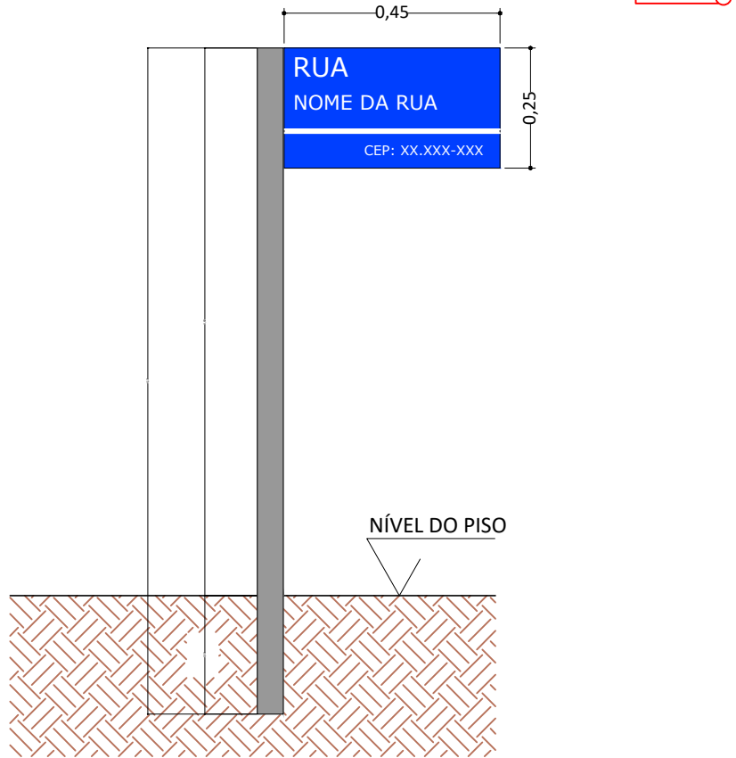
DETALHE DA PLACA DE NOME DE VIA: sem escala
